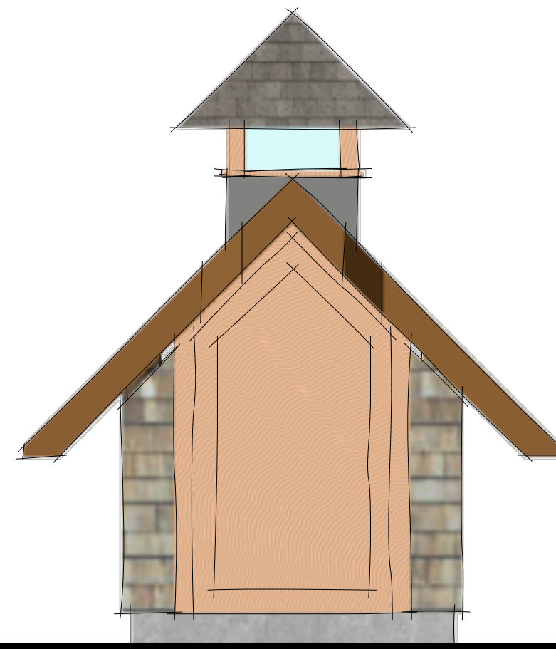
Door elevation
